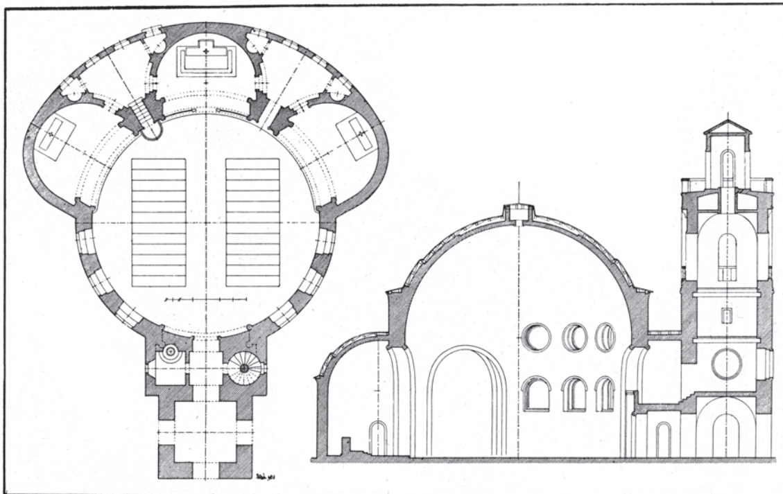
J. PLEČNIK: STUDIJA CERKVE ZA B — TLORIS IN PREREZ
