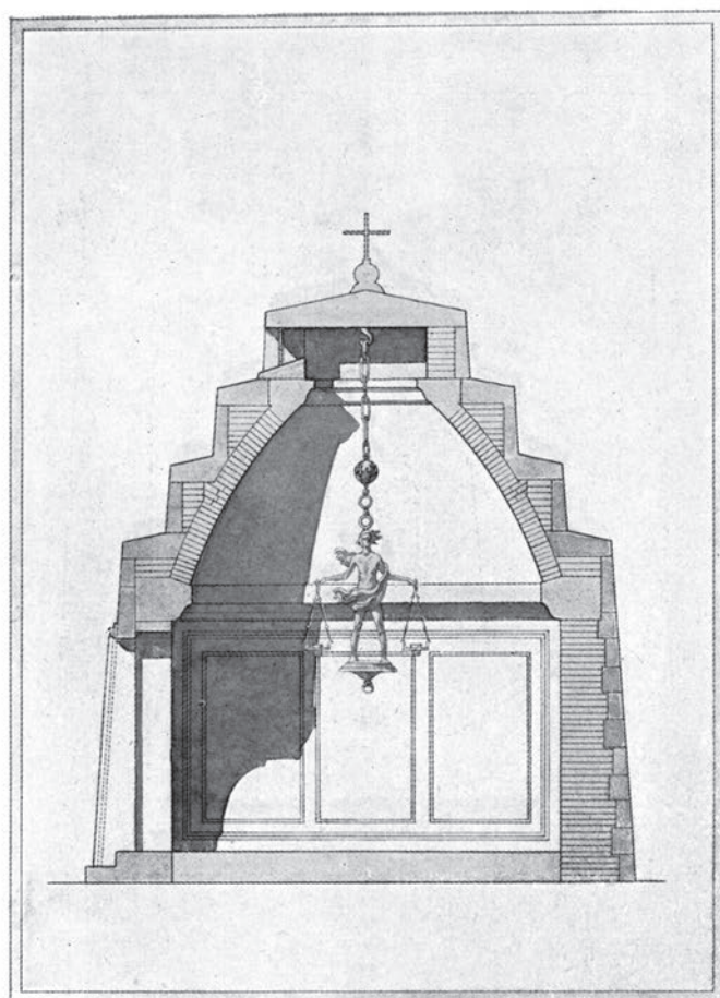
MIRKO ORAŽEM: MAVZOLEJ — PREREZ
