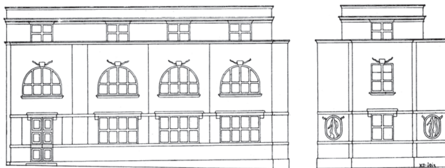
J. PLEČNIK: PRIZIDEK — FASADA
