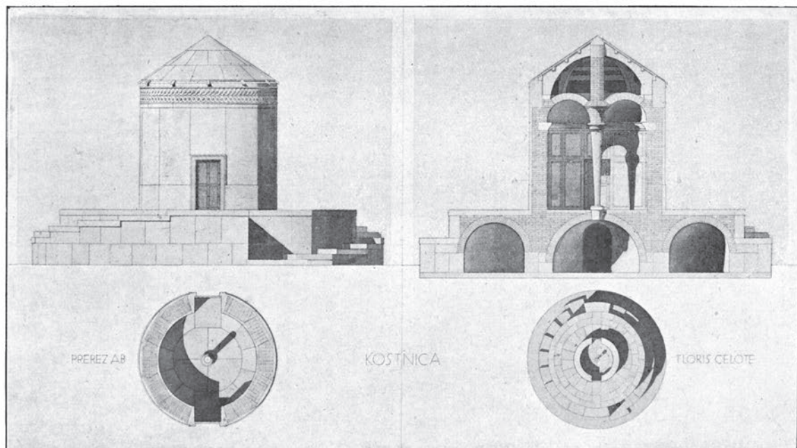
BORIS KOBE: STUDIJA KOSTNICE ZA LJUBLJANO
