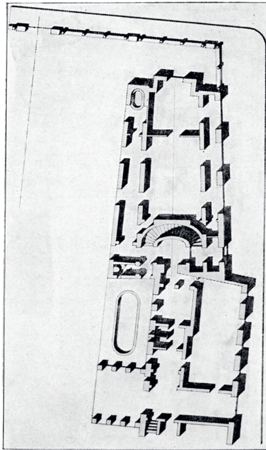
J. PLEČNIK: PRIZIDEK — TLORIS
