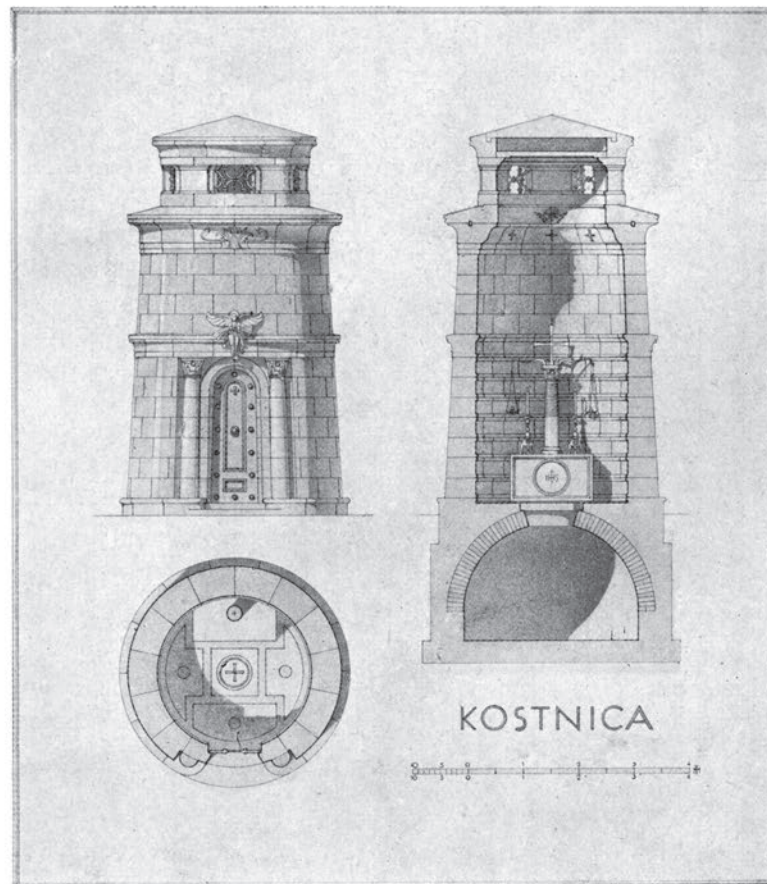
JANKO VALENTINČIČ: STUDIJA KOSTNICE
