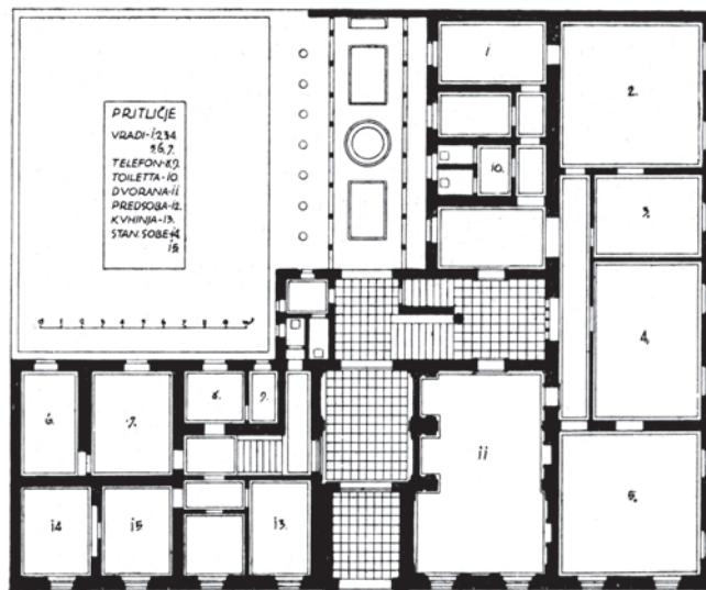
FRANCÈ TOMAŽIČ: ADAPTACIJA TRG. IN OBRT. ZBORNICE V LJUBLJANI — TLORIS
