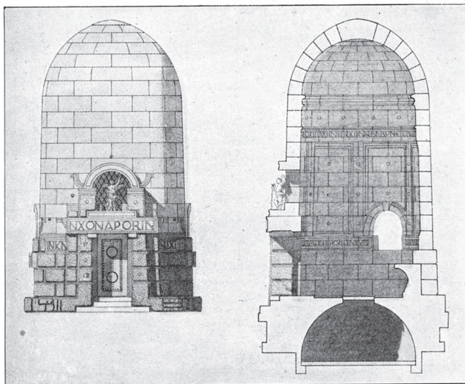
JANKO OMAHEN: STUDIJA KOSTNICE
