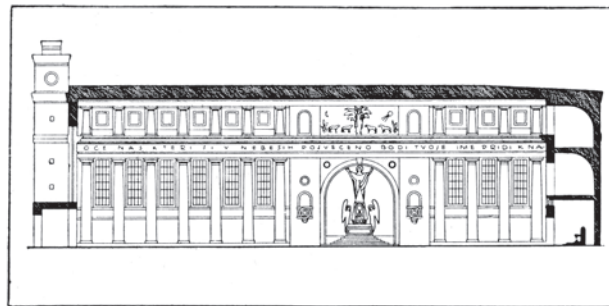
FRANCÈ TOMAŽIČ: STUDIJA Cerkve III. TLORIS IN PREREZ
