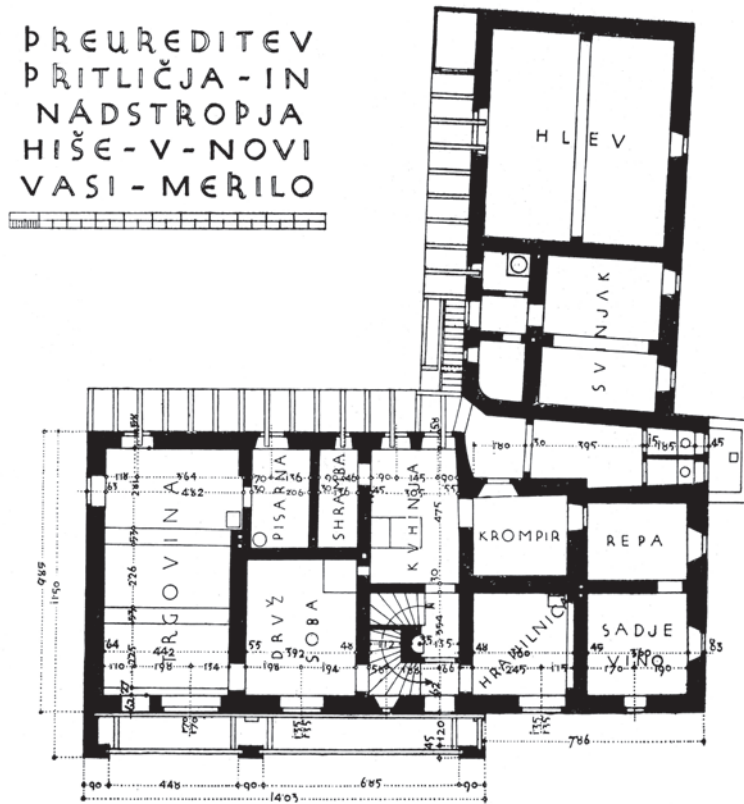
DUŠAN GRABRIJAN: PREUREDITEV HIŠE — TLORIS
