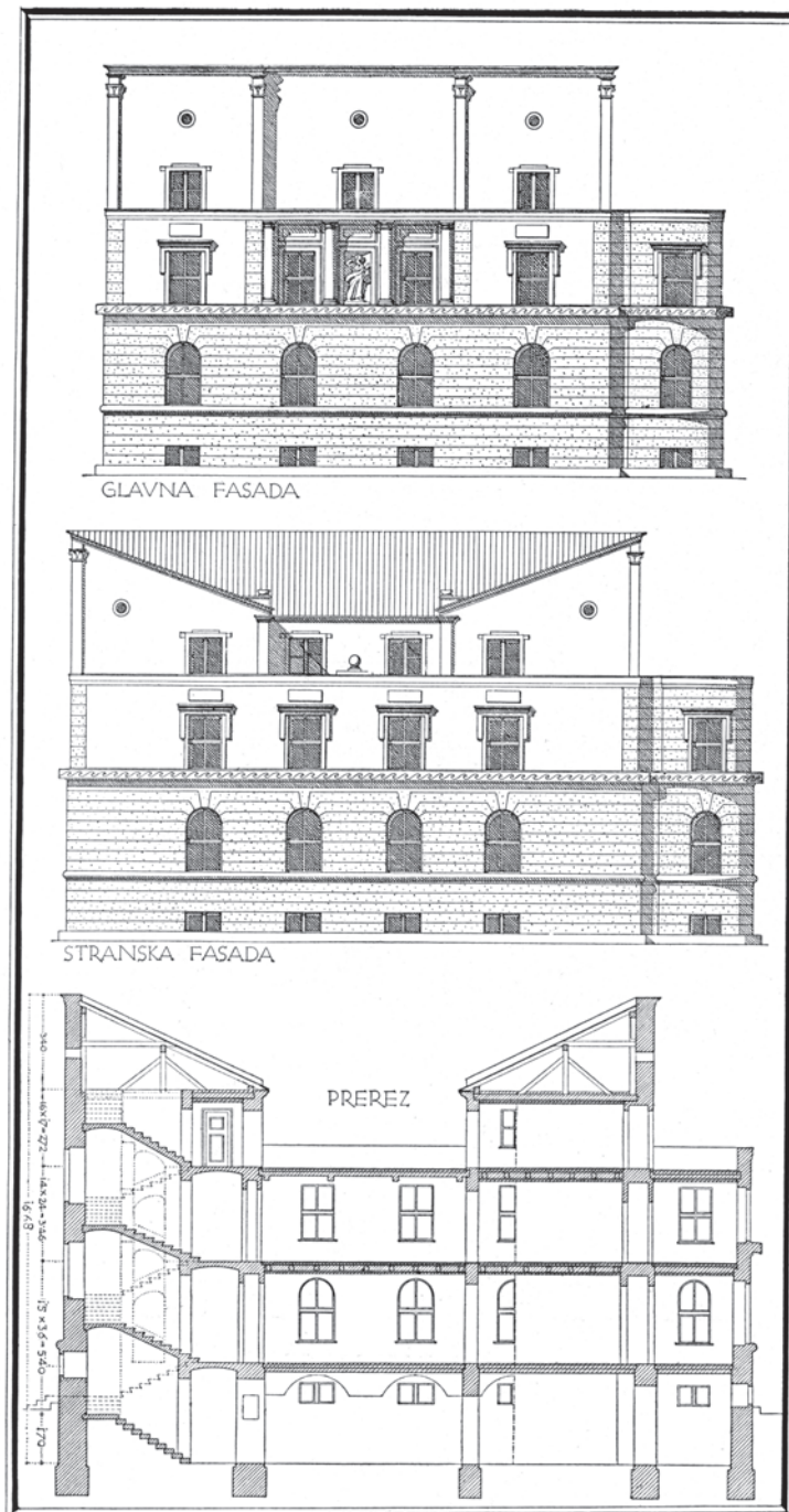
DUŠAN GRABRIJAN: DOM ARHITEKTA FASADI IN PREREZ
