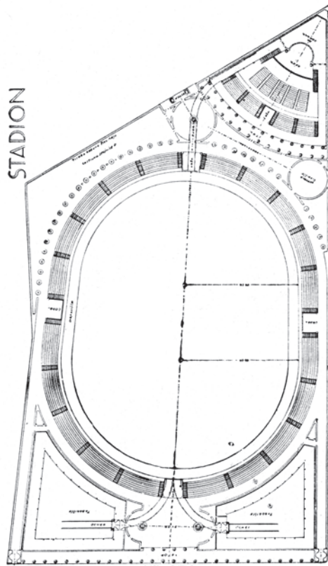
J. PLEČNIK: TLORIS STADIONA
