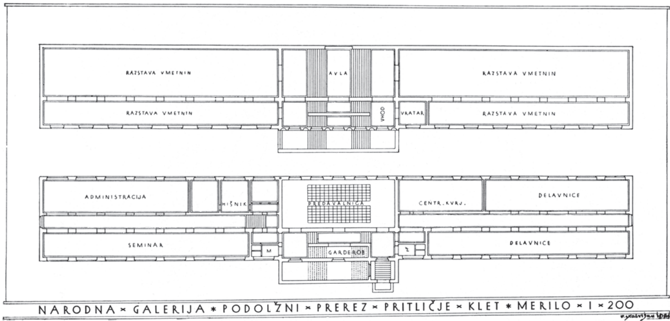
DUŠAN GRABRIJAN: TLORIS PROJEKTA NARODNE GALERIJE V REGULIRANEM PARKU TIVOLI V LJUBLJANI
