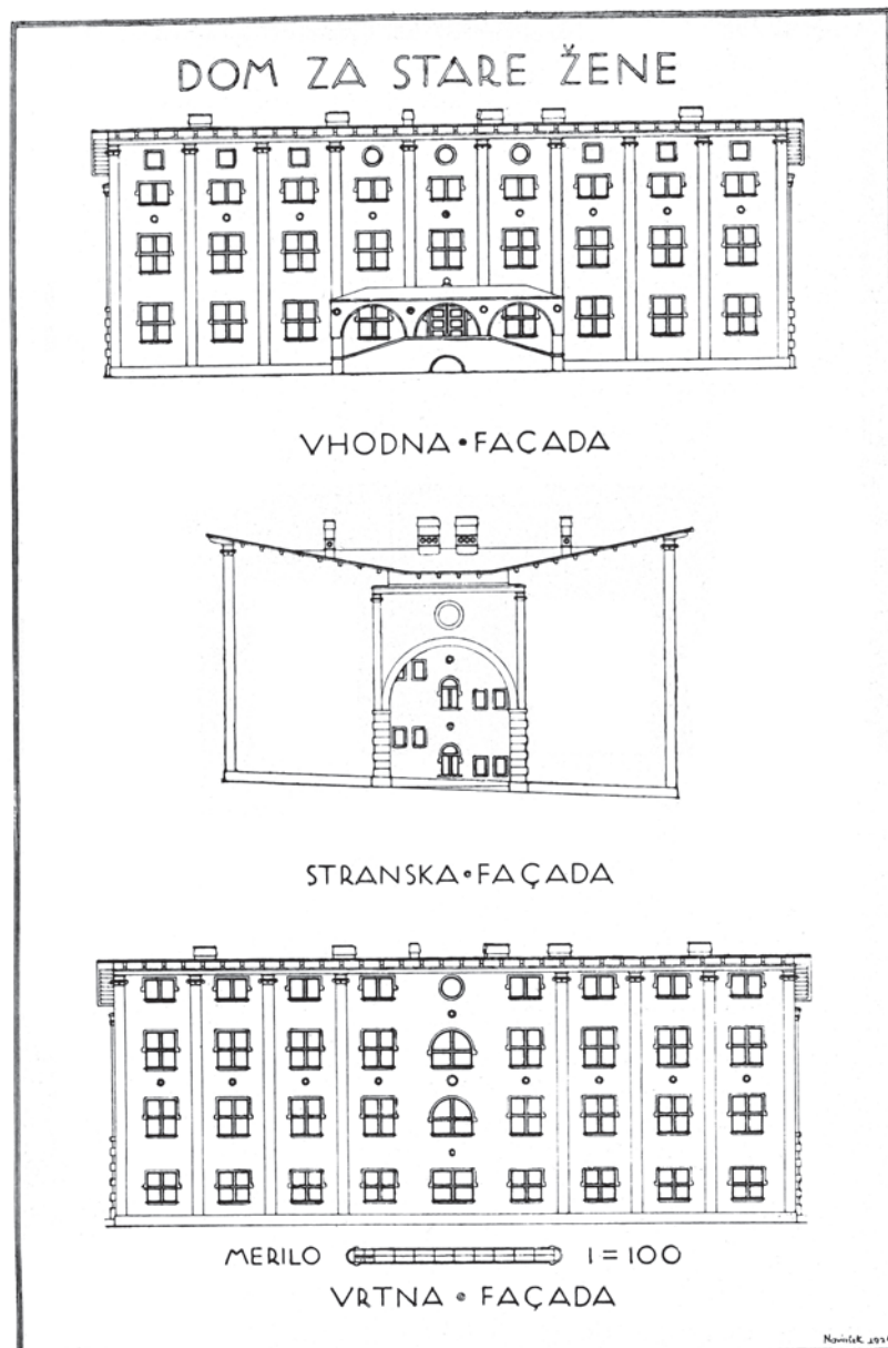
EMIL NAVINŠEK: ZAVETIŠČE SVOBODNIH — FASADE
