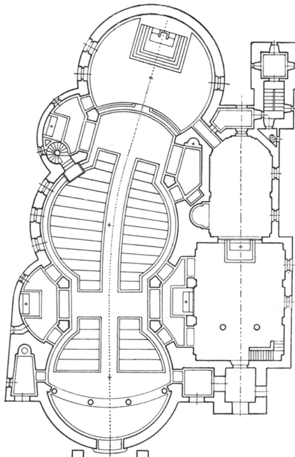
FRANČE TOMAŽIČ: STUDIJA CERKVE I. — TLORIS
