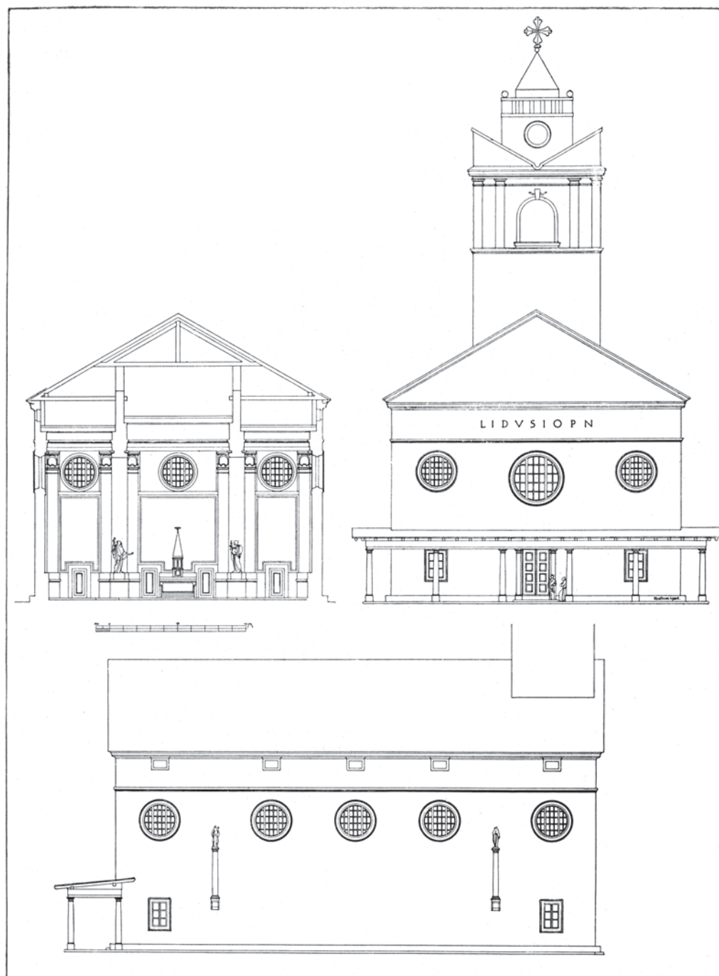
J. PLEČNIK: STUDIJA FARNE CERKVE — PREREZ IN FASADI
