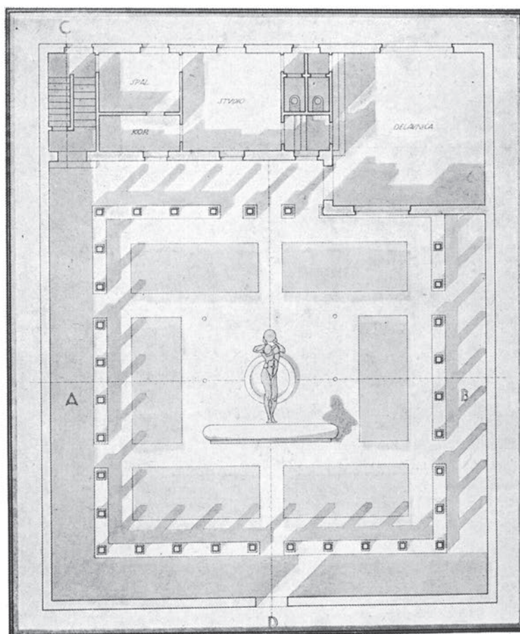
BORIS KOBE: UMETNIKOV DOM — TLORIS
