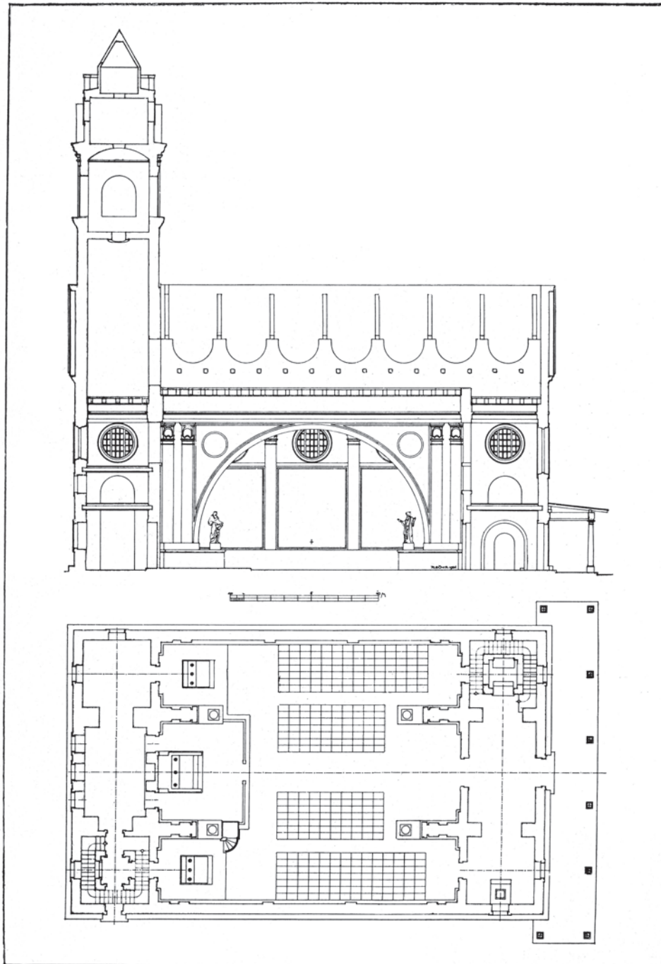
J. PLEČNIK: STUDIJA FARNE CERKVE — TLORIS IN PREREZ
