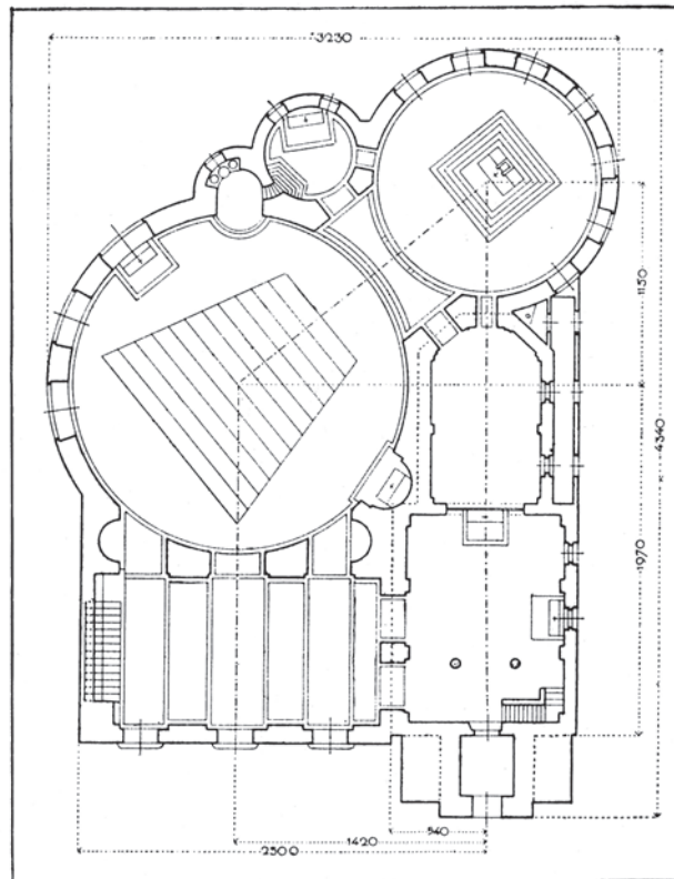
FRANCÈ TOMAŽIČ: STUDIJA Cerkve II. TLORIS
