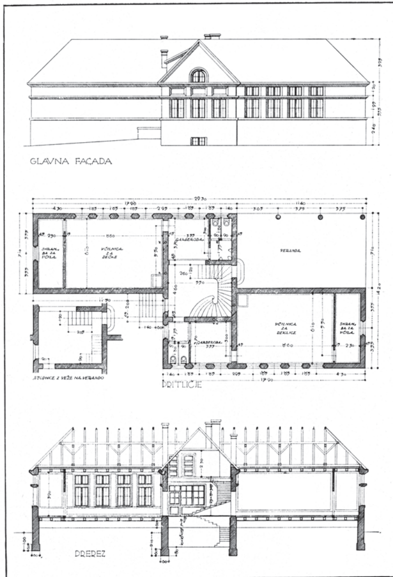
JAROSLAV ČERNIGOJ: DVORAZREDNA ŠOLA
