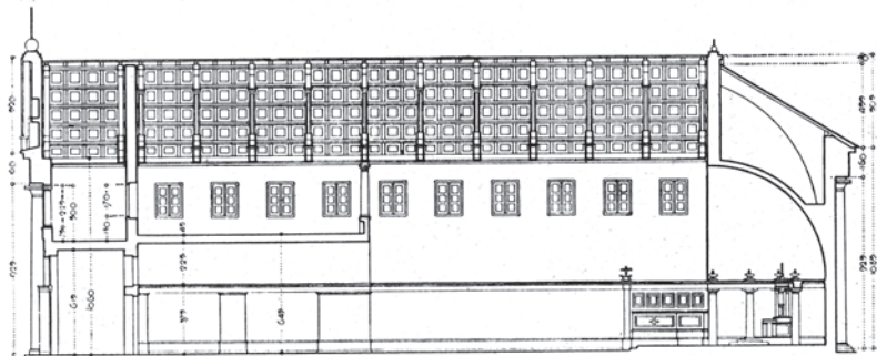
POGLED NA PEVSKI KOR
