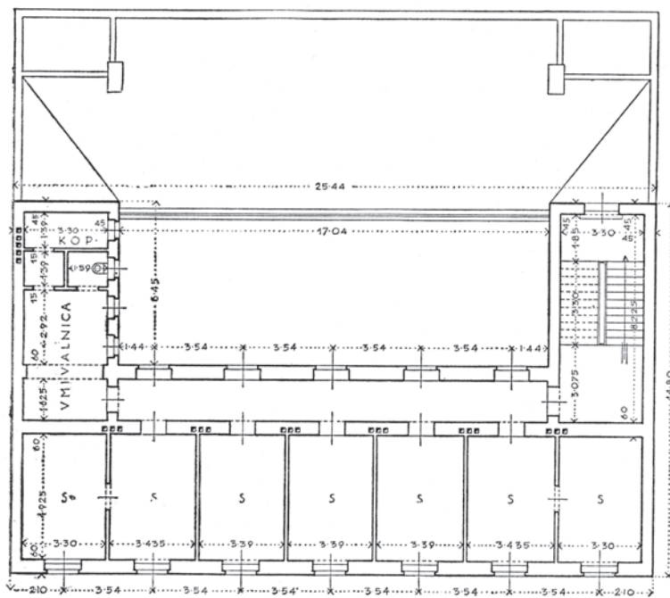
DRUGO NADSTROPJE
