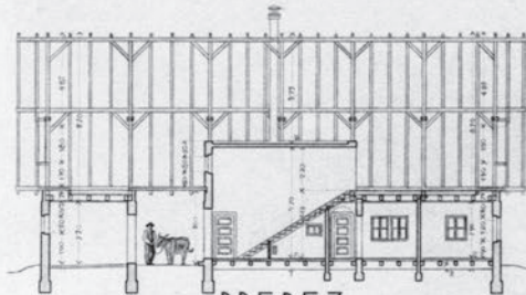
PREREZ
