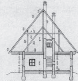
PREREZ
