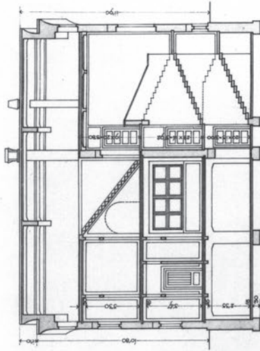
PREREZ A-B
