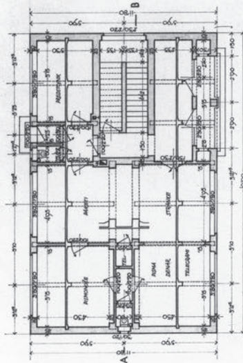
PRITLICIE
