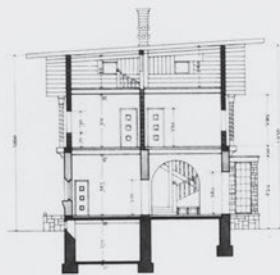
REZ V-V
