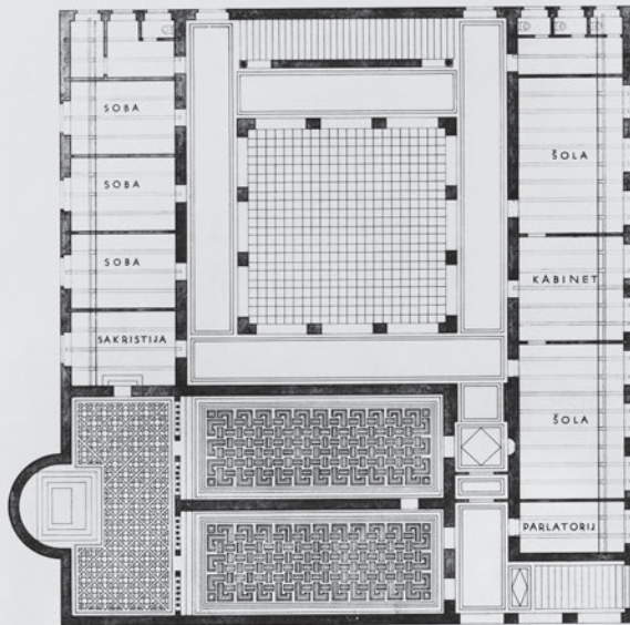
PRITLIČJE
