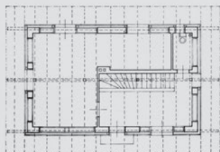
NADSTROPJE
