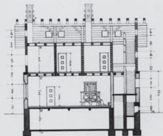
REZ I-I
