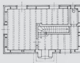
PRITLIČJE
