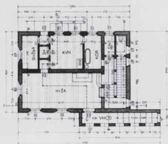
PRITLIČJE
