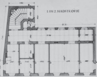
PRVI ET
